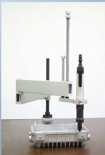
電動/氣動鎖入工具 共用之手臂
