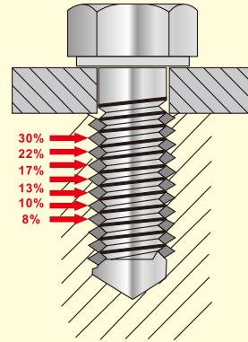
使用Powercoil護套後的螺絲
